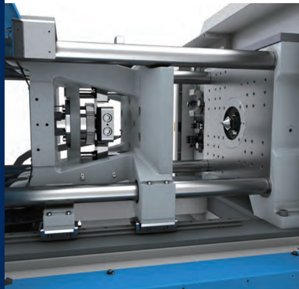
双重线性导轨支撑提供最佳的模板平行度
